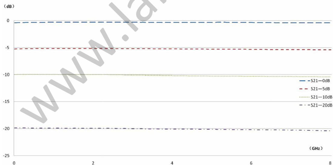
衰减值测试曲线 Attenuation Test Curve
